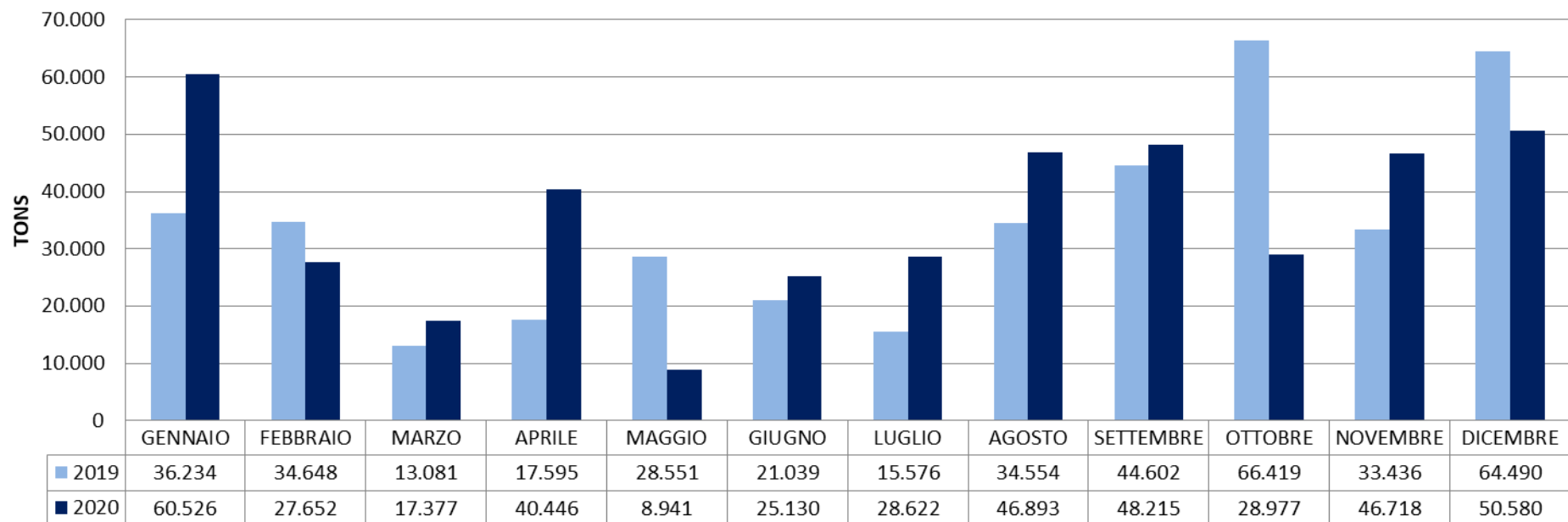
PORTO DI MANFREDONIA - ANDAMENTO DELLA MOVIMENTAZIONE DELLE RINFUSE SOLIDE PER MESE - CONFRONTO ANNI 2019 2020
