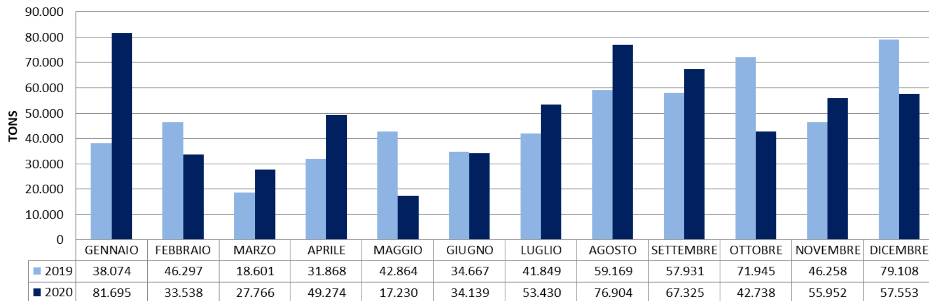
PORTO DI MANFREDONIA- ANDAMENTO DELLA MOVIMENTAZIONE DEL TOTALE TONNELLATE MERCI PER MESE CONFRONTO ANNI 2019 2020
